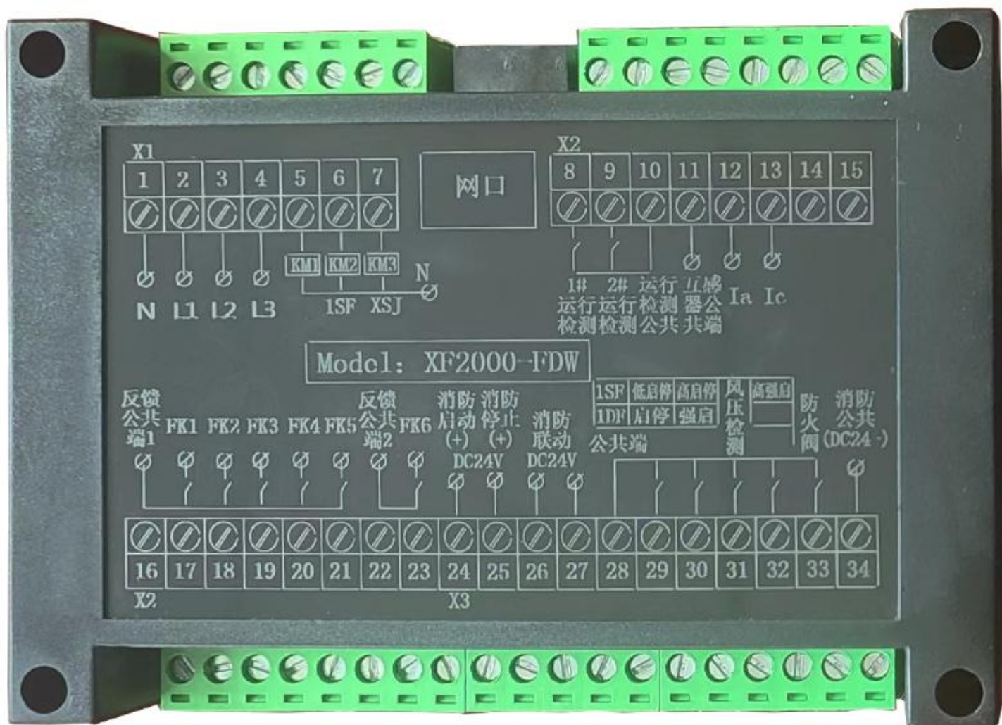
控制器底壳尺寸 145*90*40mm
